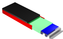
Opbouw flexibele afstandhouder
